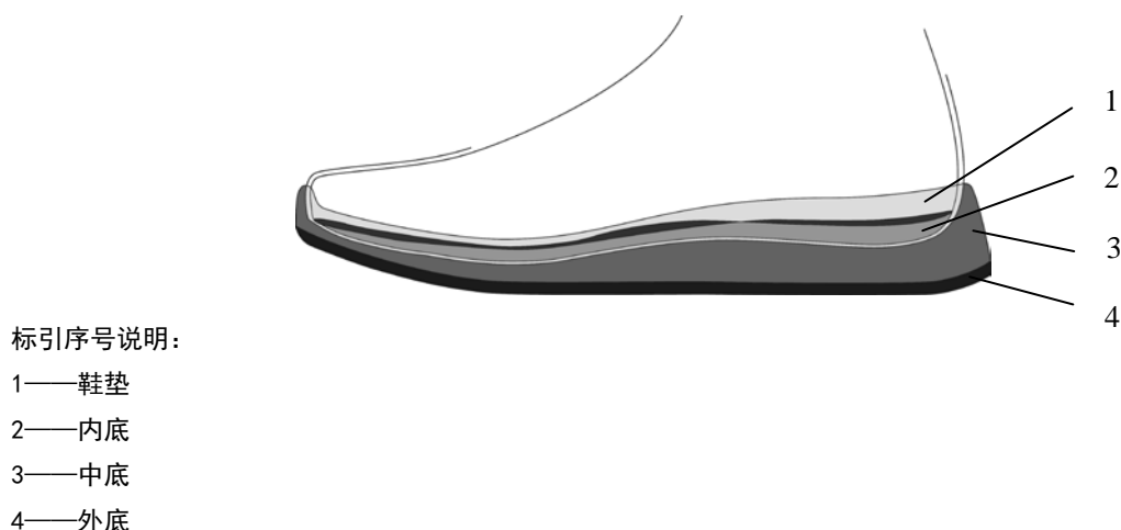
图10 鞋底结构示意图
